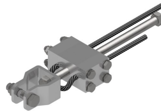
Seilklemme Typ A 8 mm
